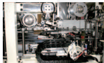
粘着フィルム貼付け装置
