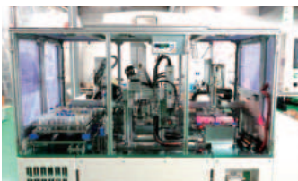
自動分注装置
